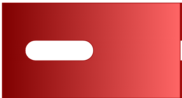
L spojka s oválnou dírou 80x42x2mm slitina AlMgSi 0,5
