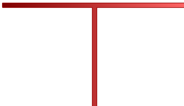
T profil 80x45x2mm slitina AlMgSi 0,5
