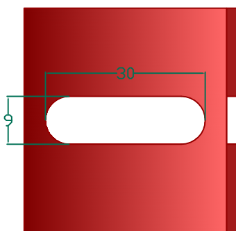
L spojka s oválnou dírou 42x42x2mm slitina AlMgSi 0,5
